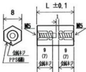
PS5A (M5 P-0.8)
