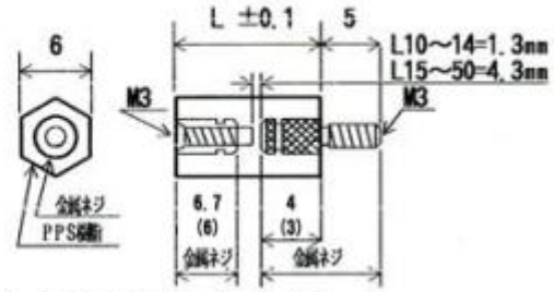
PS3B (M3 P-0.5)
