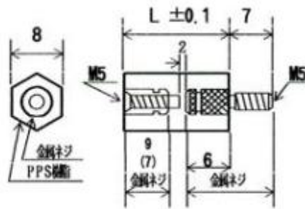
PS5B (M5 P-0.8)
